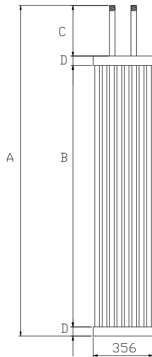
Modello EST 35 a 8 tubi
