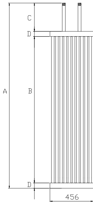
Modello EST 45 a 10 tubi
